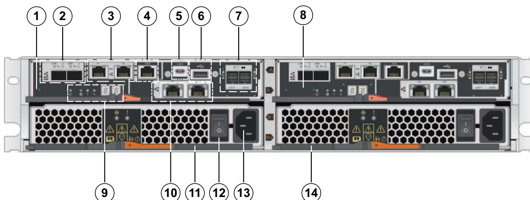
Блок с двумя контроллерами на 12 отсеков — вид сзади
