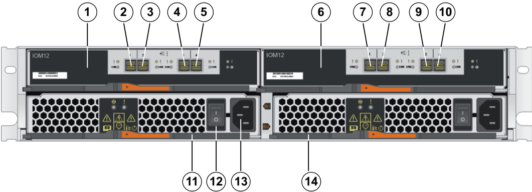
Блок расширения на 12 отсеков – вид сзади
