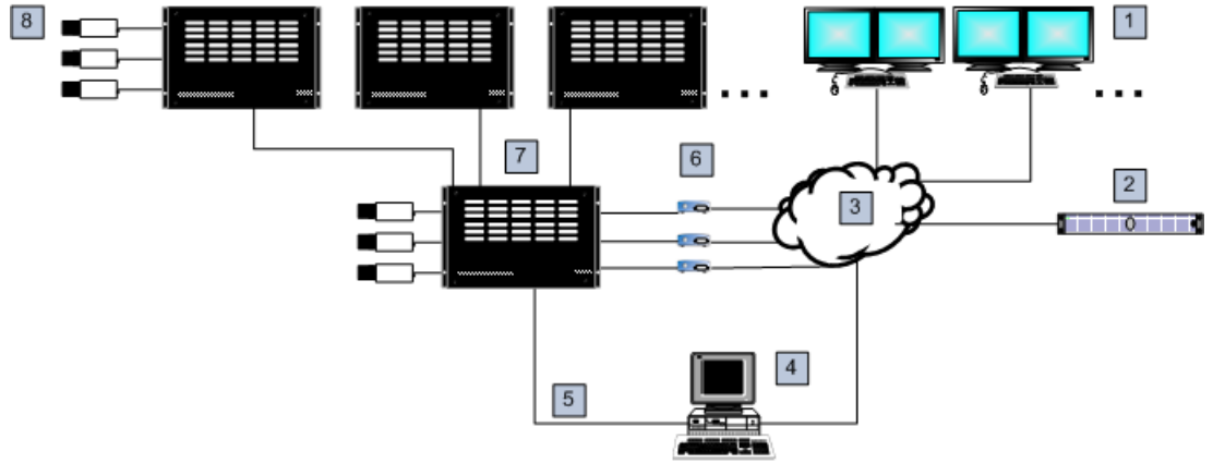
Şekil 5.1: Satellite anahtarlarıyla genişletilmiş Bosch Allegiant sistemi
