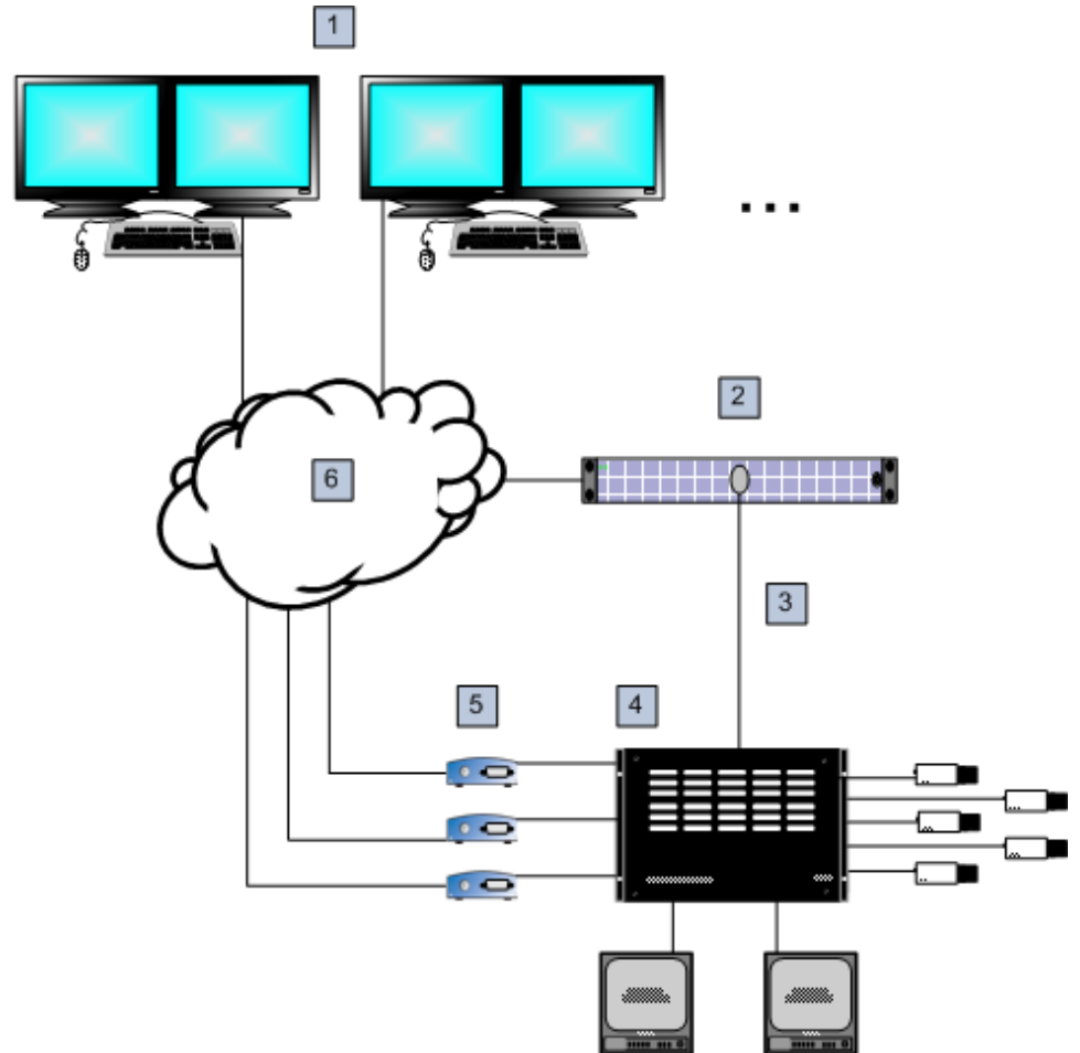
Şekil 5.1: Bosch Video Management System'in Bosch Allegiant matris anahtarına yerel bağlantısı
