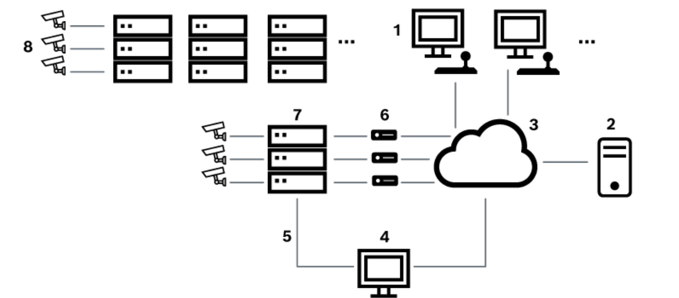
Attēls 6.5: Bosch Allegiant sistēma, kas paplašināta ar satelīta slēdžiem
