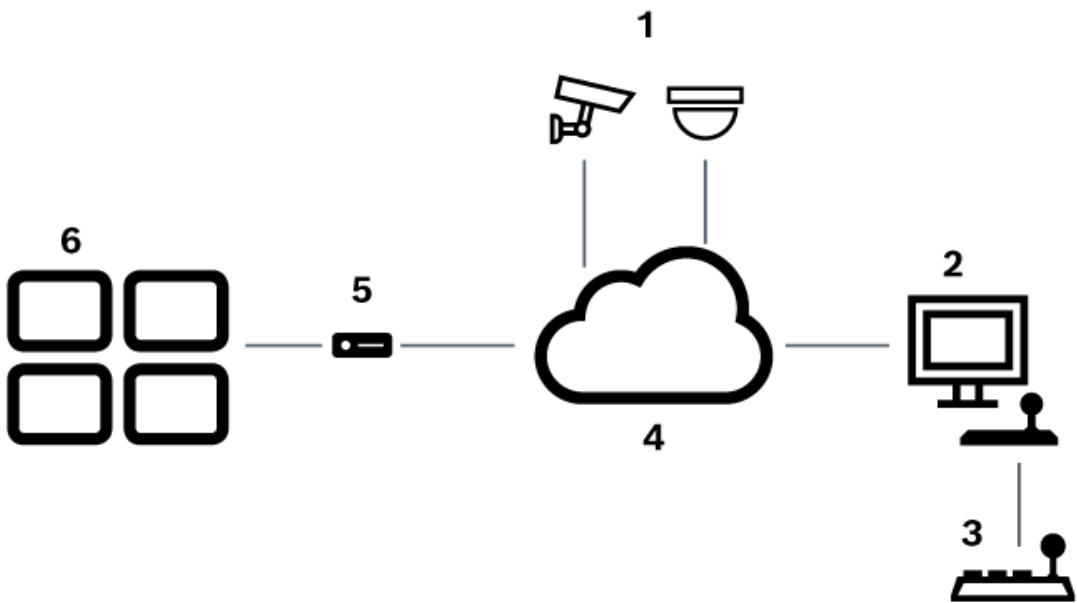
Figure 6.1: Scénario 1 : clavier IntuiKey de Bosch connecté à un poste de commande Bosch Video Management System
