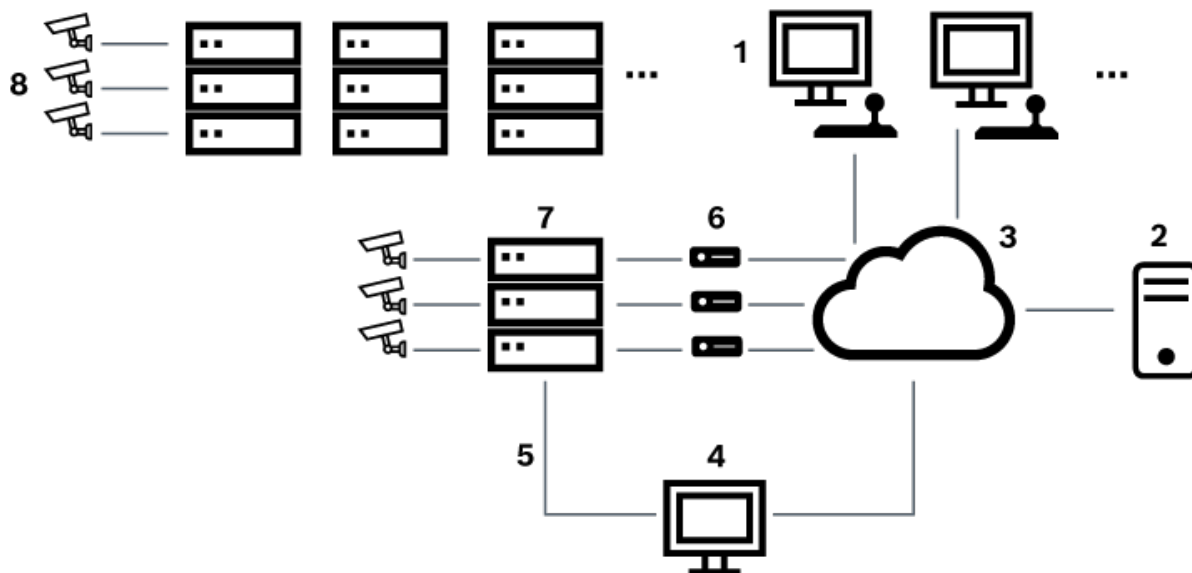
Figure 6.5: Système Bosch Allegiant étendu à l'aide de systèmes de commutation satellites
