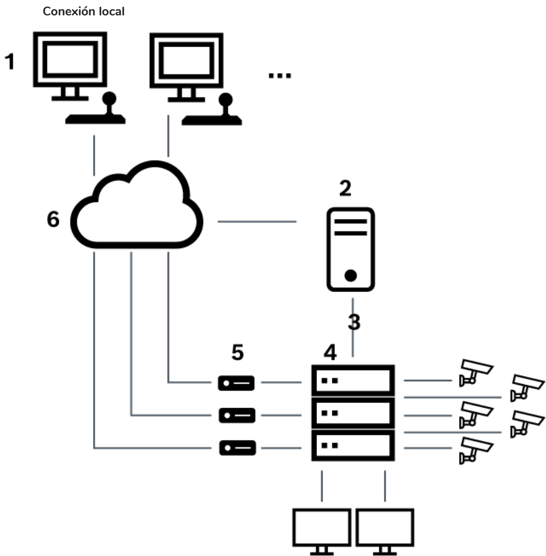
Figura 6.3: Conexión local de Bosch Video Management System a una matriz Allegiant de Bosch
