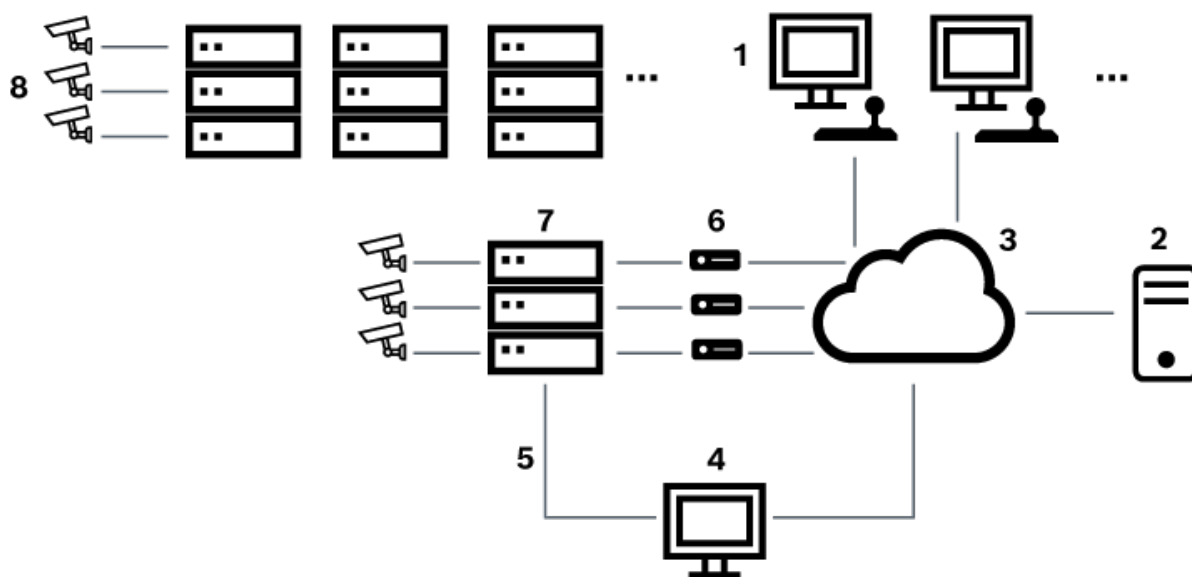
Figura 6.5: Sistema Bosch Allegiant ampliado con matrices satélite
